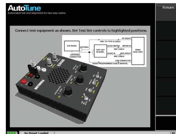
XTSオートチューン・セットアップ図
